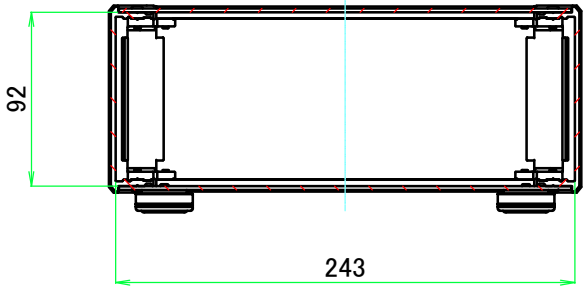
A-A ( 1 : 4 )
