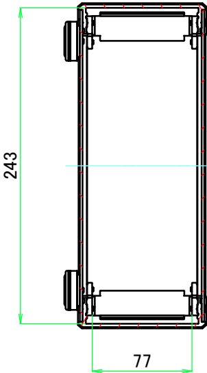
B-B ( 1 : 4 )
