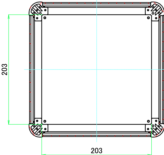
C-C ( 1 : 4 )
